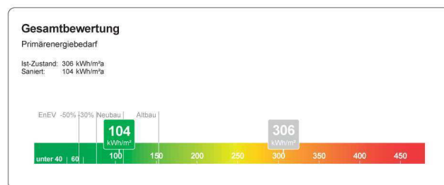
Reihenendhaus von 1970: Energiebedarf vorher - nachher.
